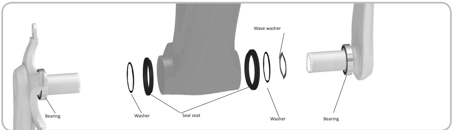
Figure 14.24. Campagnolo bearing set
